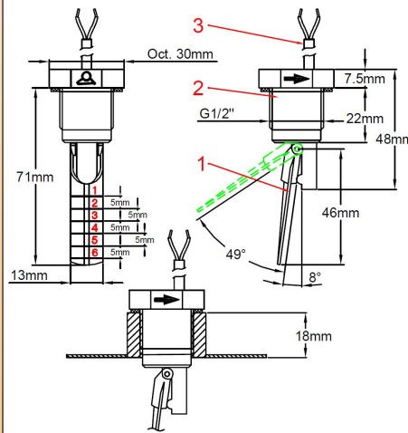
1: Palette 2: Corps 3: Cable R1S (½"BSPP)
